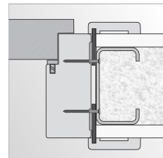
montáž na vruty do stěny ze sádrokartonu
